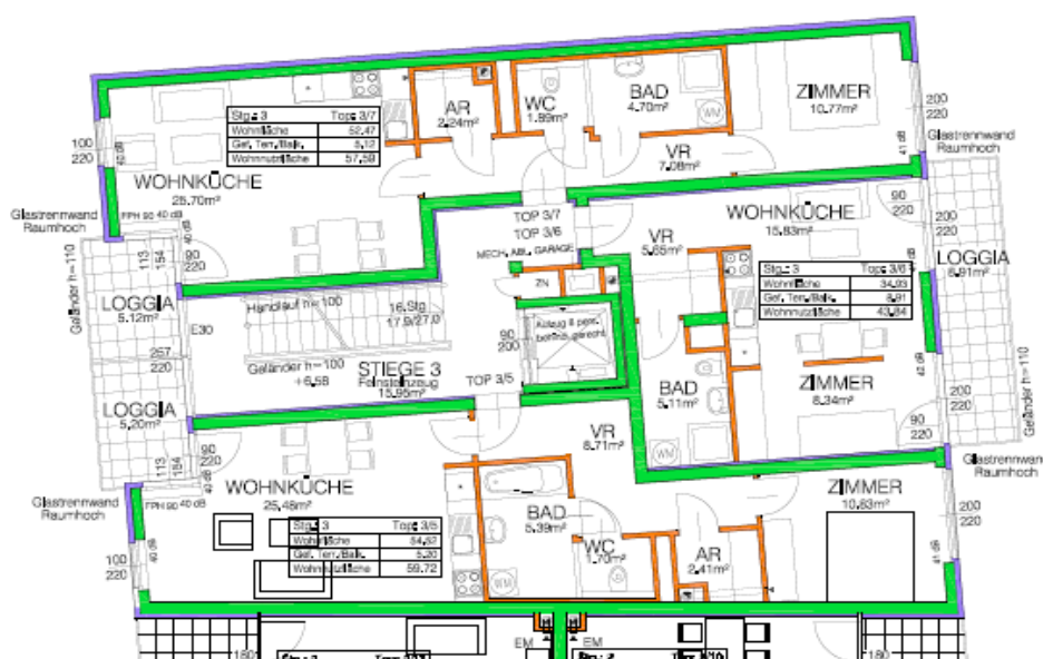
Abb.: Grundrisstypen „Hofhaus“
